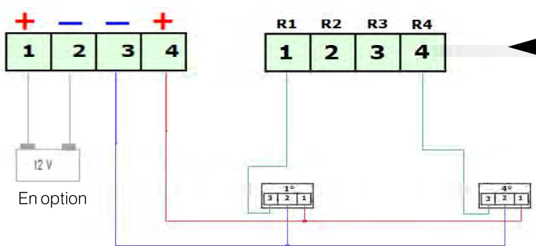
Connexion des sondes et d'éventuelle batterie
