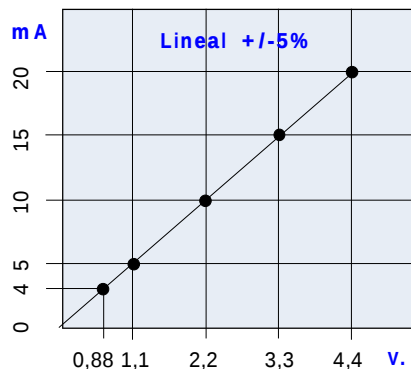
Grafico de conversión corriente / tensión con resistencia de carga de 220 \Omega
