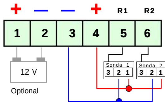
Conexión de las sondas y eventual batería
