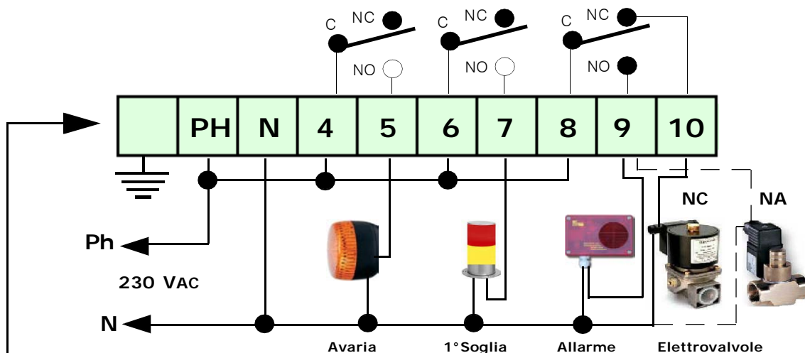
Collegamenti di una Elettrovalvola Normalmente Chiusa senza Sicurezza Positiva inserita
