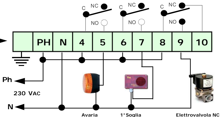
Alimentazione centralina e collegamento di una Elettrovalvola con sirene a 12 VDC, tramite una fonte alternativa, e ricarica batteria
