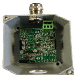
Sonde avec capteur démonté
