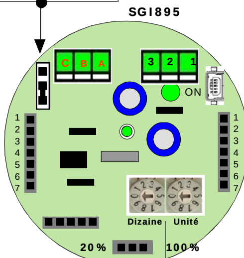
Commutateurs d'adressage
