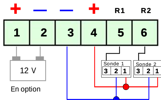
Connexion des sondes et d'éventuelle batterie
