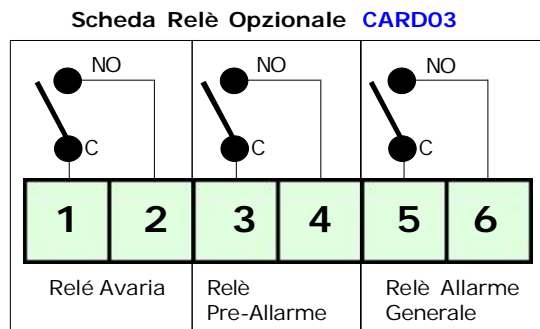
Collegamento TS1008
