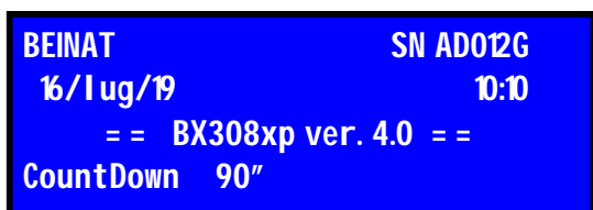
Schermata che appare all'accensione della BX308xp . Questa schermata rimane accesa 90 secondi.
